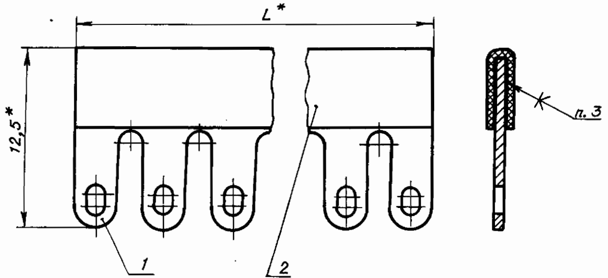
Размеры, мм
