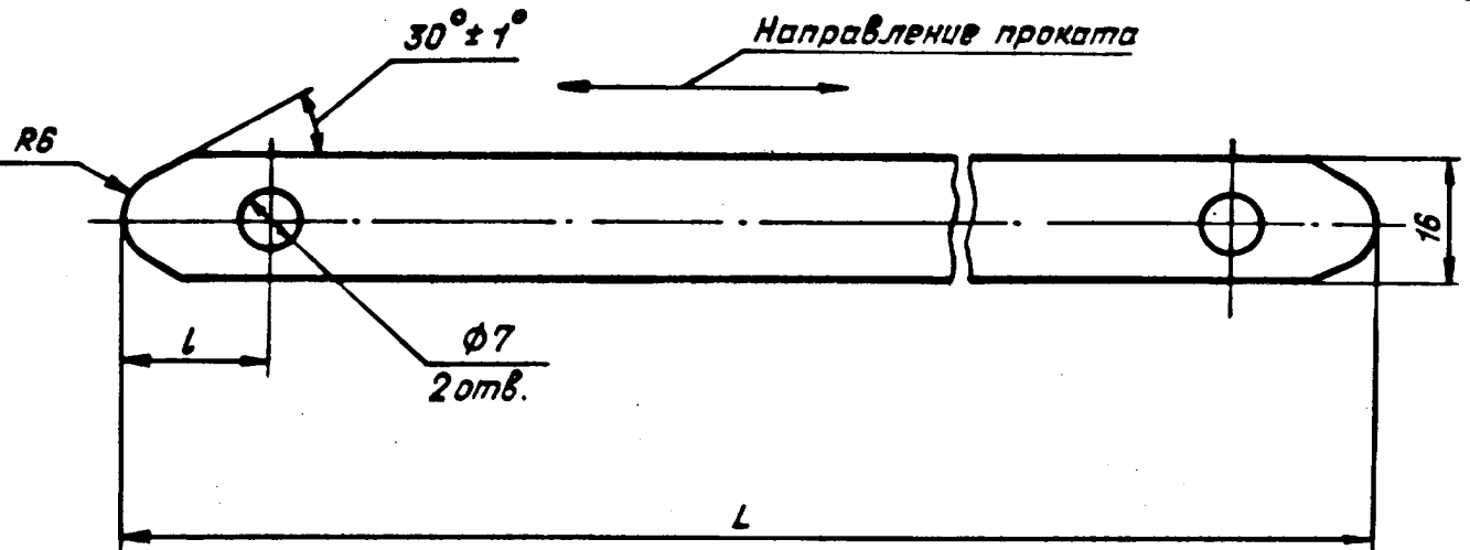
Развертка
