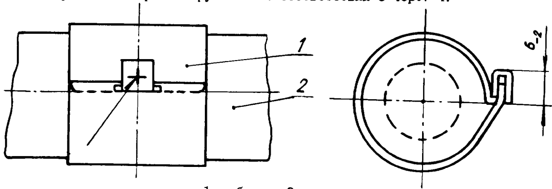
1 - бирка; 2 - рукав
