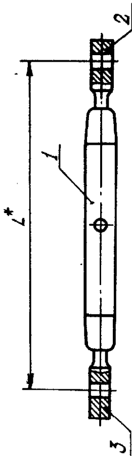
Размеры, мм
