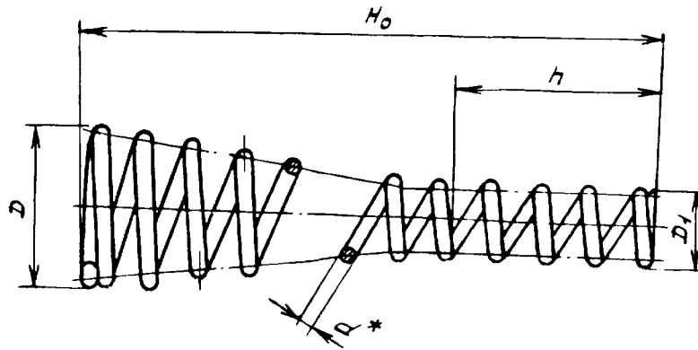
Размеры, мм
