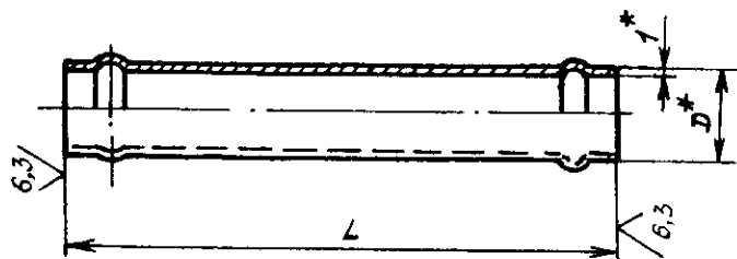
Размеры, мм
