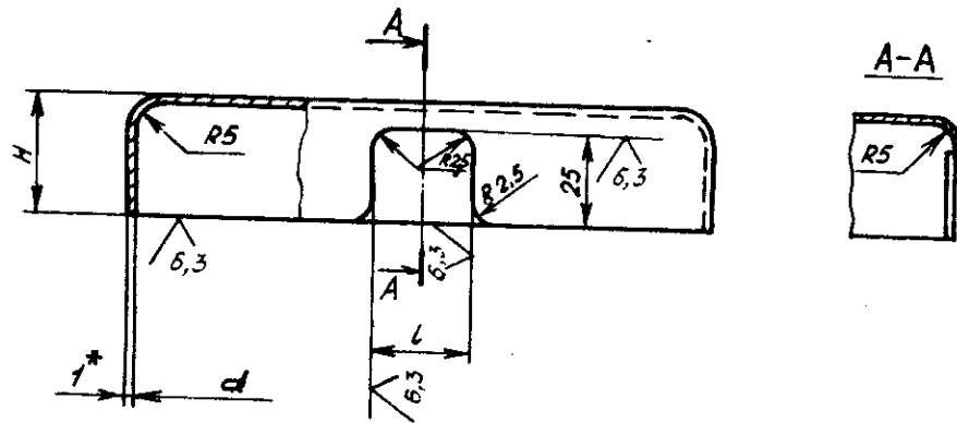
Размеры, мм
