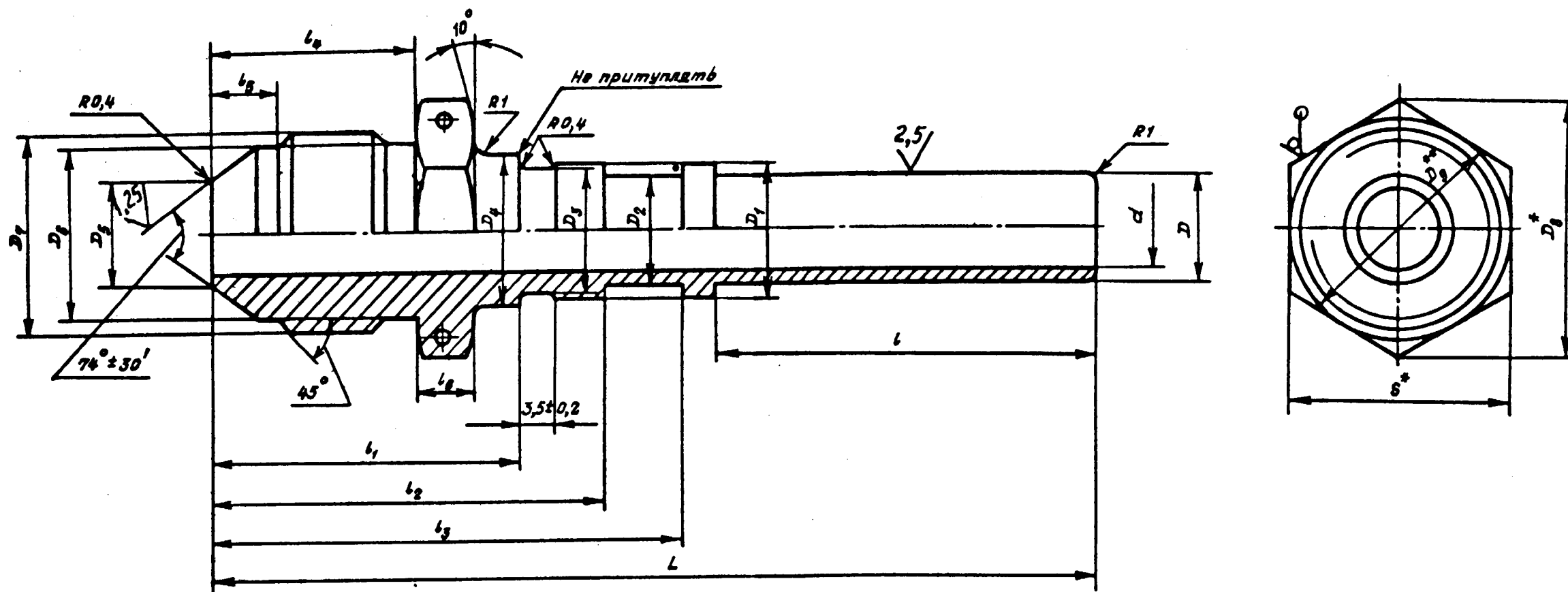
Размеры, мм
