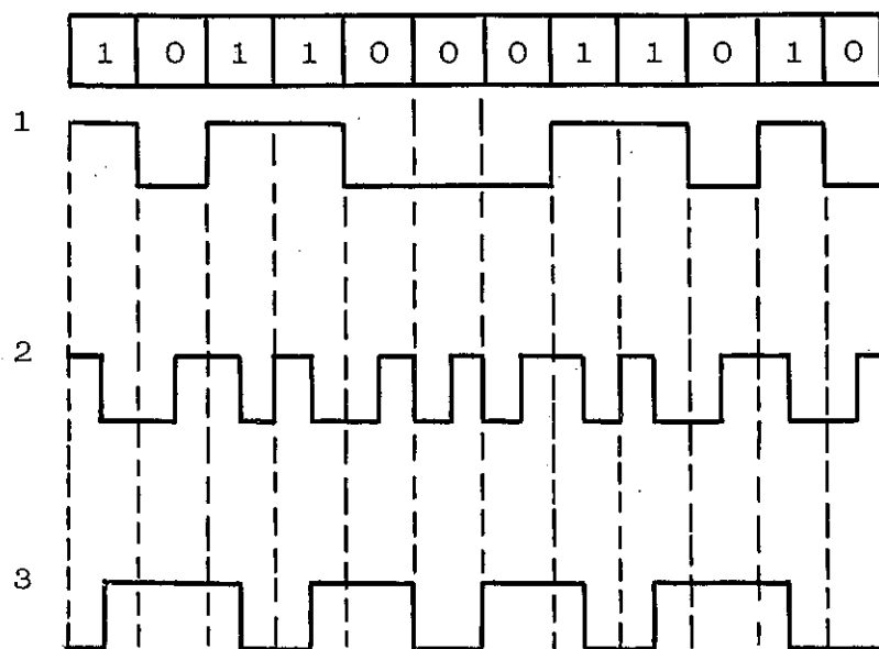
Последовательность бит
