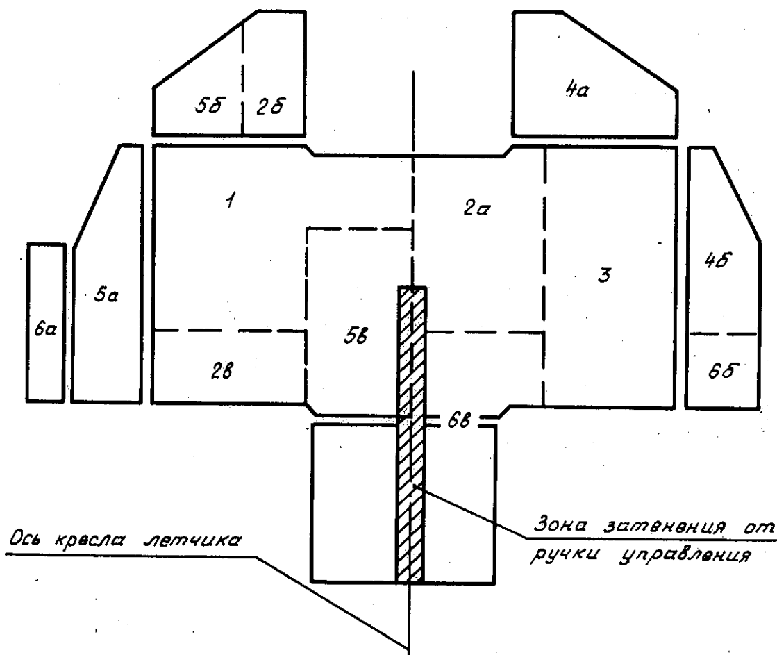
Зоны приборной доски летчика учебно-тренировочного самолета
